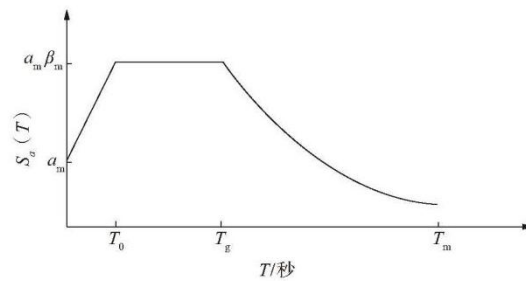
图 B.1 加速度反应谱的形式
